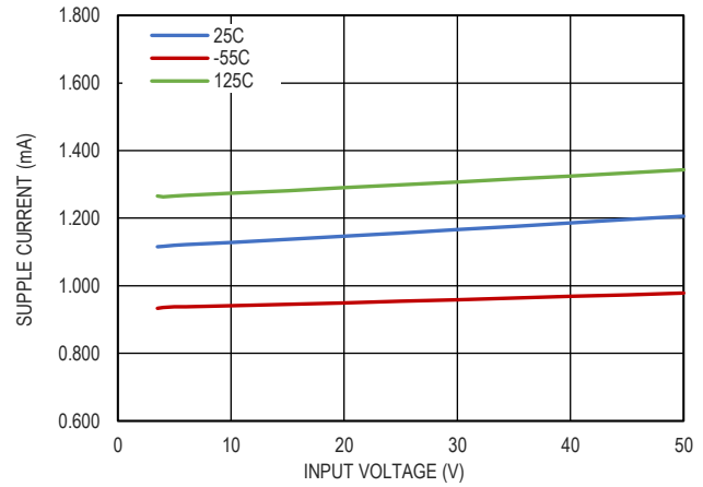
图 18. 输入电流和输入电压的关系, V_{OUT}=2.048V
