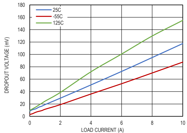
图 22. 最小输入电压和输出电压的关系, V_{OUT}=4.096V
