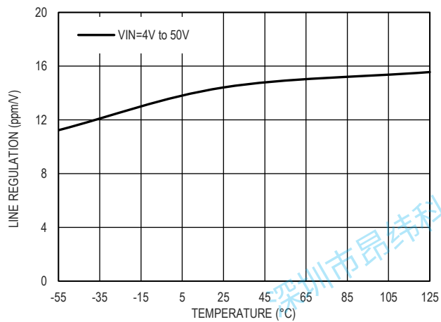
图 13. 输入调整率和温度的关系, V_{OUT}=1.25V
