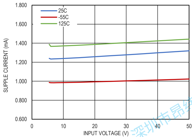
图 19. 输入电流和输入电压的关系, V_{OUT}=3.3V
