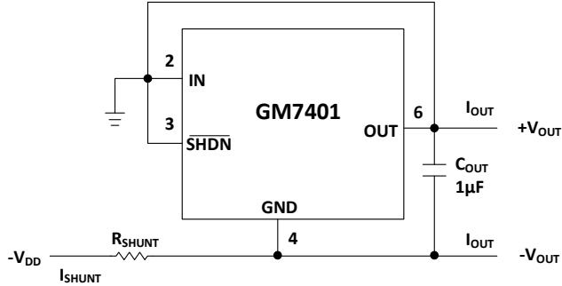
图 26. 负压并联方式
