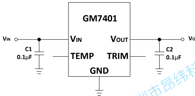
图 23. 有电容的应用电路
