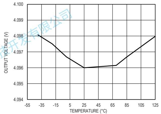
图 8. 4.096V 输出电压和温度的关系
