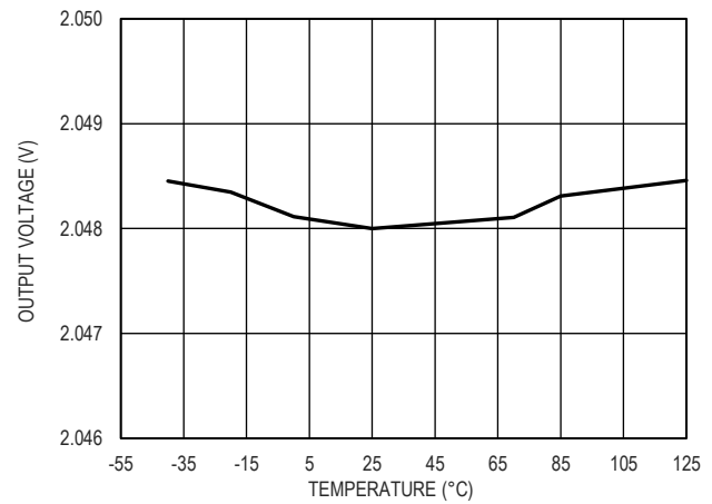
图 6. 2.048V 输出电压和温度的关系
