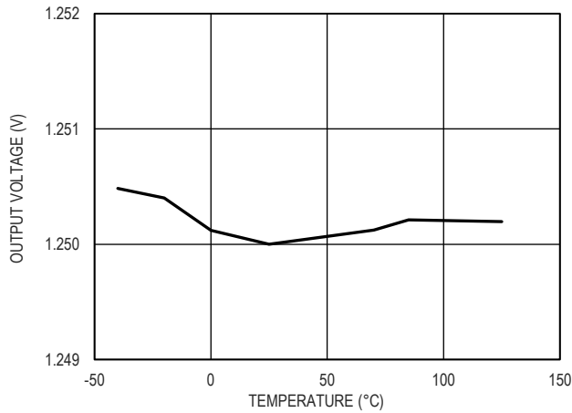
图 5. 1.25V 输出电压和温度的关系
