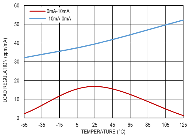
图 9. 负载调整率和温度的关系, V_{OUT}=1.25V
