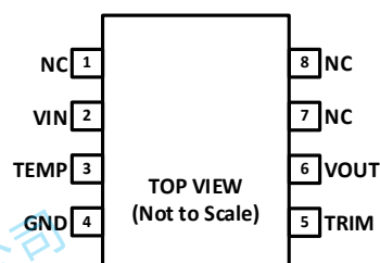
图 2. 8 引脚 SOIC
