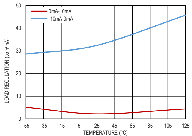
图 10. 负载调整率和温度的关系, V_{OUT}=2.048V
