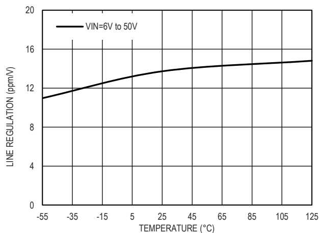
图 15. 输入调整率和温度的关系, V_{OUT}=3.3V
