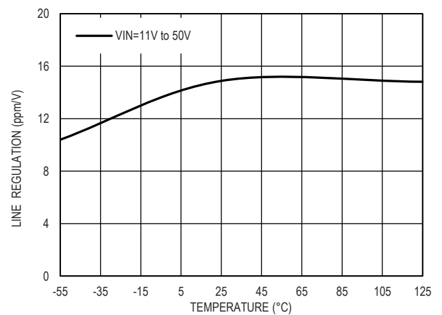
图 16. 输入调整率和温度的关系, V_{OUT}=4.096V
