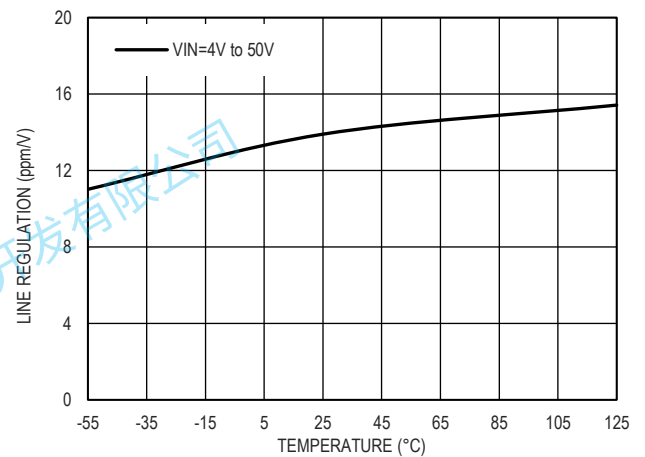
图 14. 输入调整率和温度的关系, V_{OUT}=2.048V
