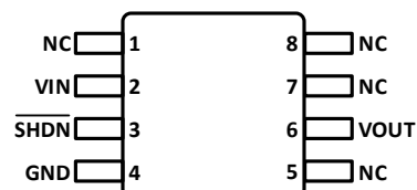
图 1. 8 引脚 MSOP
