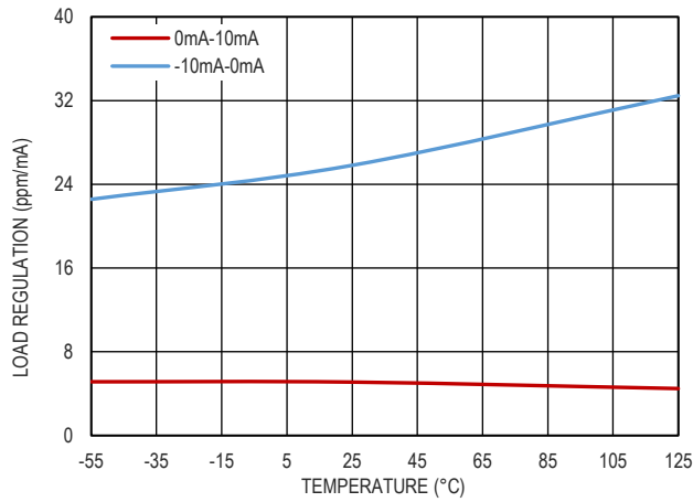
图 11. 负载调整率和温度的关系, V_{OUT}=3.3V
