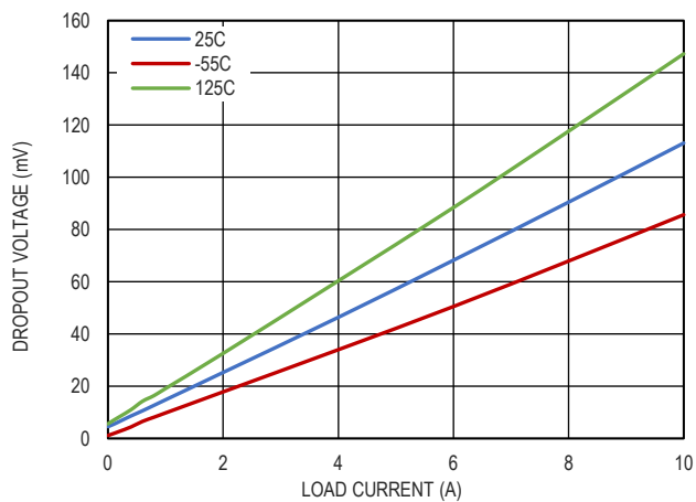
图 21. 最小输入电压和输出电压的关系, V_{OUT}=3.3V
