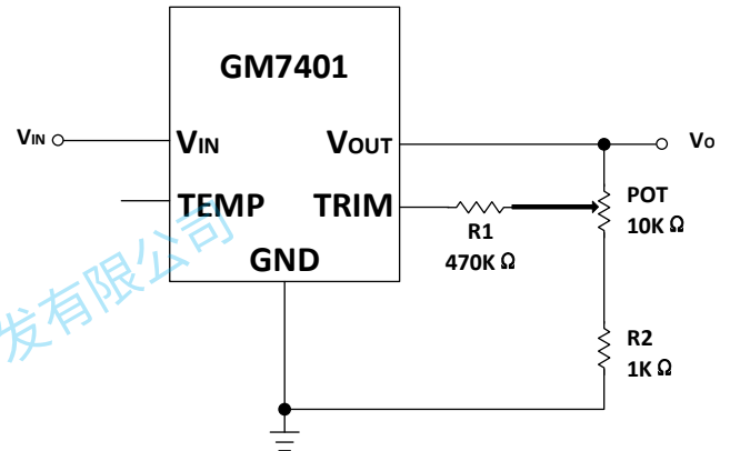
图 24. 输出电压微调电路
