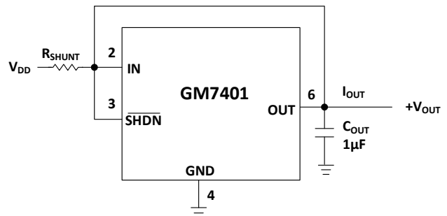
图 25. 正压并联方式
