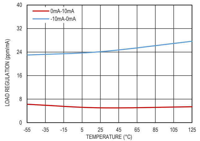
图 12. 负载调整率和温度的关系, V_{OUT}=4.096V
