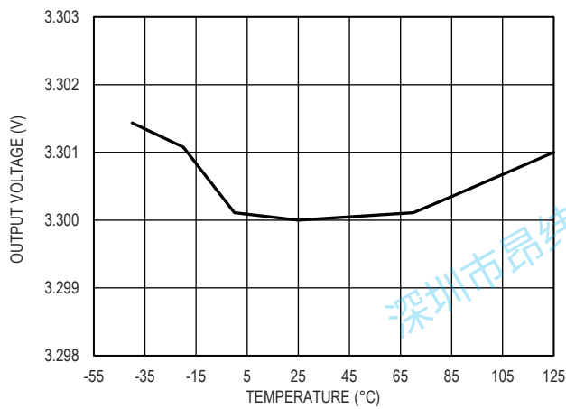
图 7. 3.3V 输出电压和温度的关系
