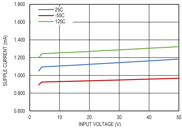
图 17. 输入电流和输入电压的关系, V_{OUT}=1.25V
