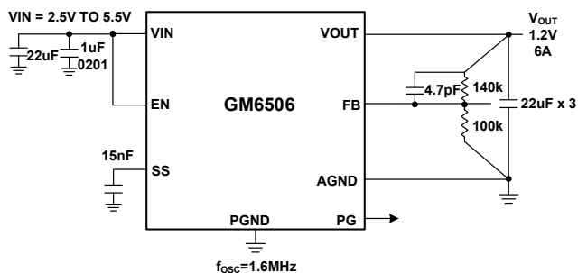
图 1. GM6506 典型应用
