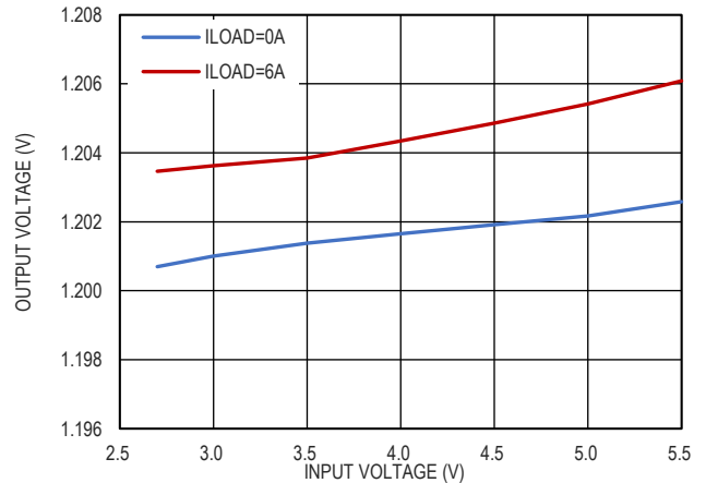
图 9. 输出电压线调整率, V_{OUT} = 1.2V
