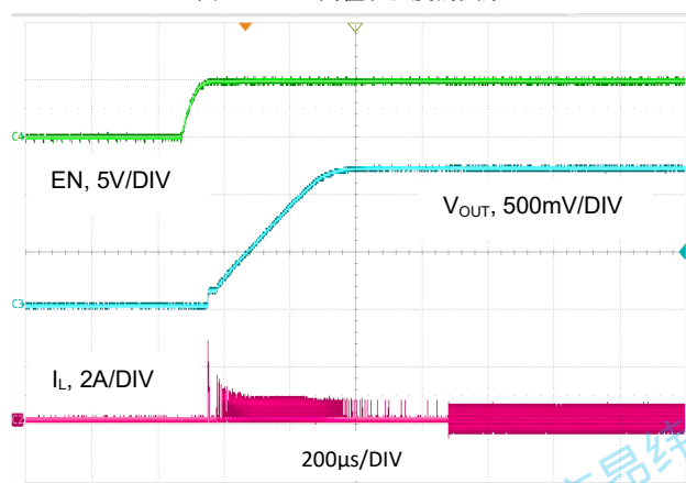
图 12. 启动波形, V_{OUT} = 1.2V , I_O = 10mA
