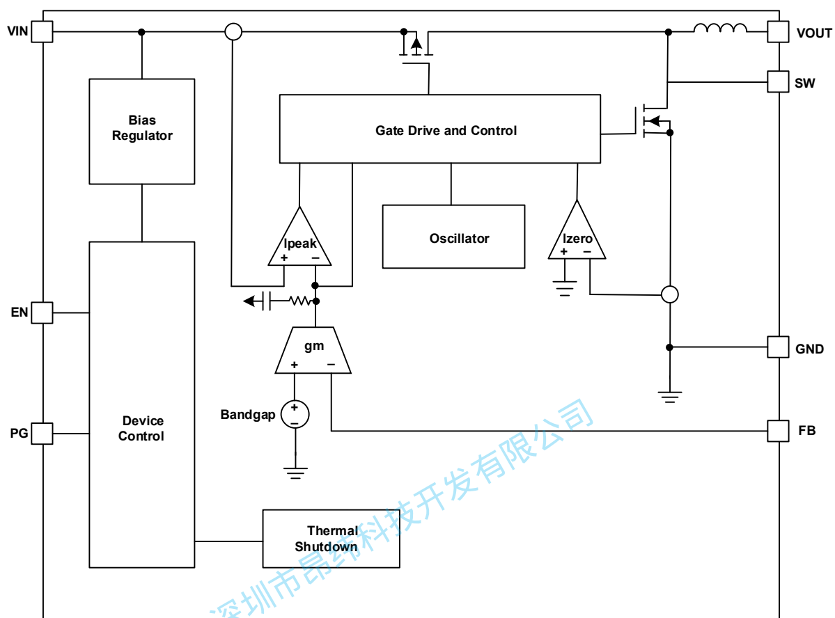
图 2 GM6506 功能框图
