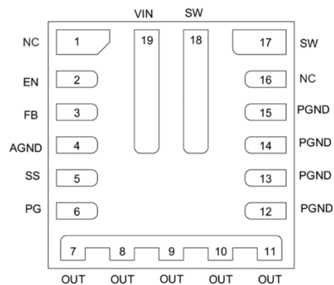
图 3 引脚配置
