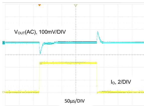
图 15. V_{OUT} = 1.2V , I_O = 0.1A 至 4.5A , FPWM 模式
