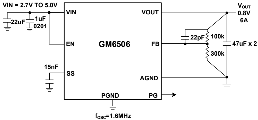
图 17. V_{IN}=3.3\text{V} , V_{OUT}=0.8\text{V} , I_{LOAD}=6\text{A}
