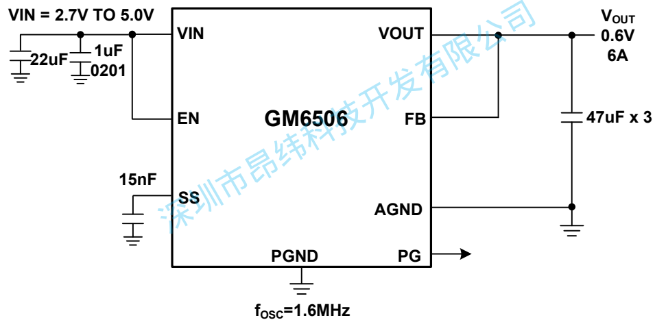
图 18. V_{IN}=3.3\text{V} , V_{OUT}=0.6\text{V} , I_{LOAD}=6\text{A}
