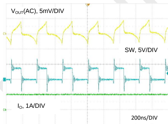
图 14. V OUT = 1.2V, I O = 1A, FPWM 模式
