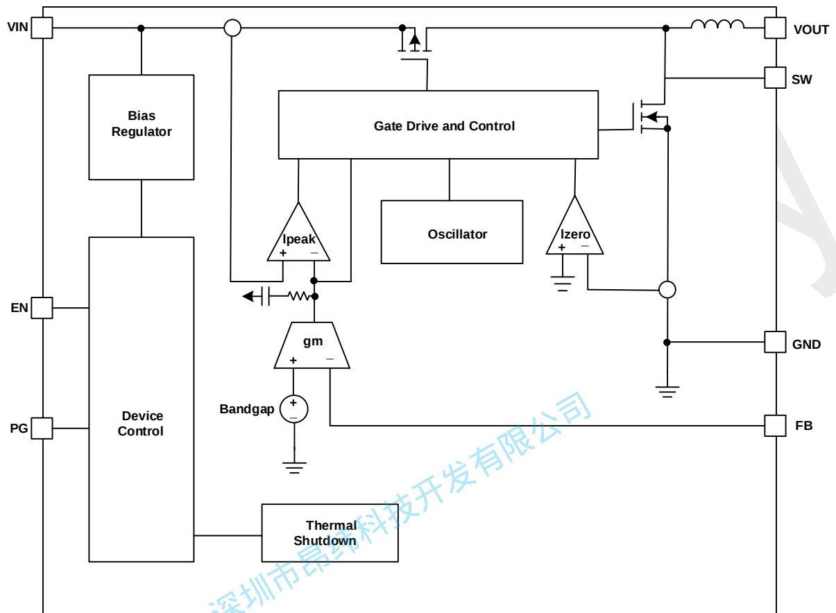
图 2 GM6504 功能框图
