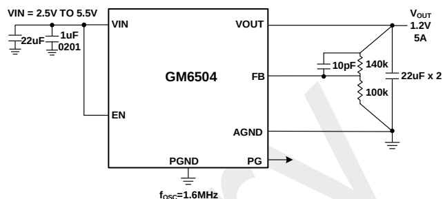
图 1. GM6504 典型应用
