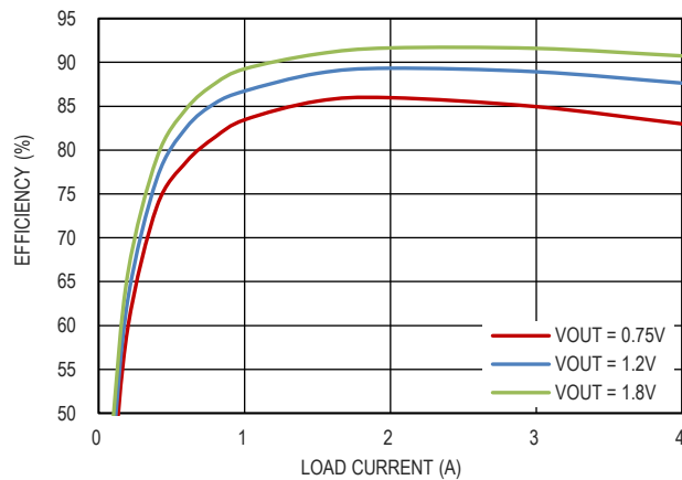
图 5. 效率曲线, V_{IN} = 5V , 低功耗模式
