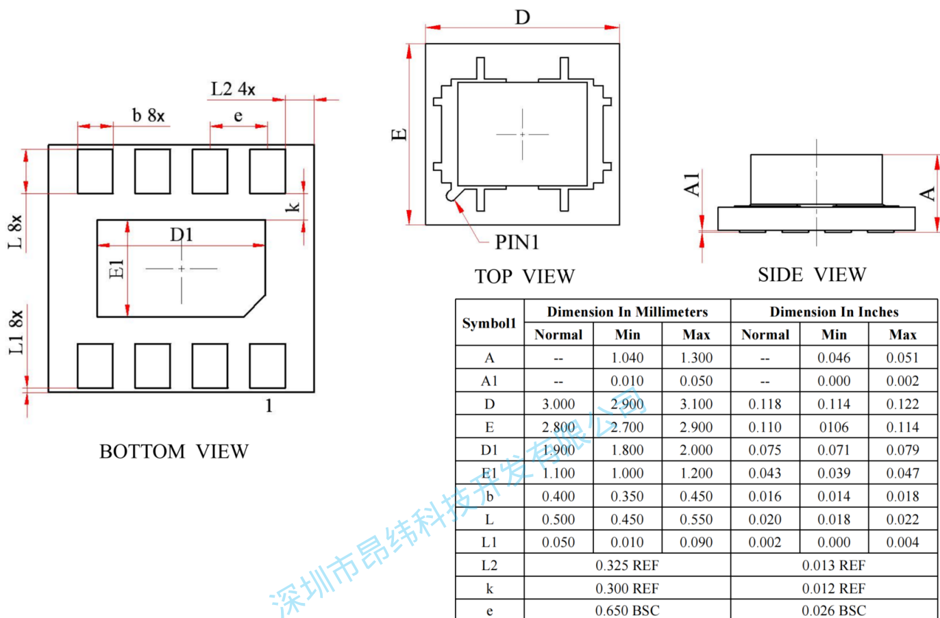
图 18.8 引脚 LGA (2.8mm x 3.0mm)
