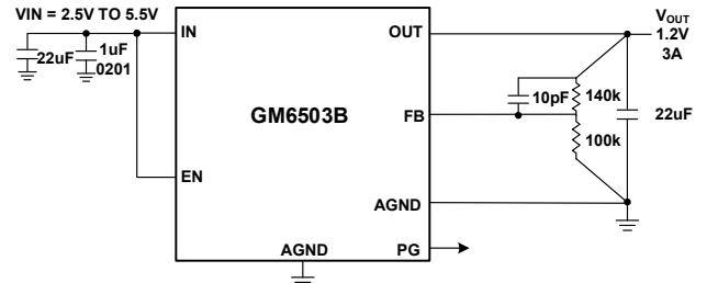
图 1. GM6503B 典型应用
