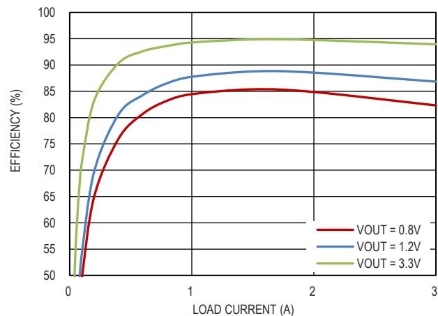
图 5. 效率曲线, V_{IN} = 5V
