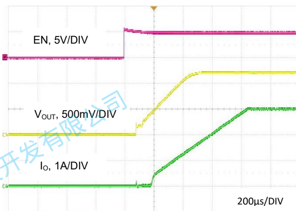
图 13. 启动波形, V_{OUT} = 1.2\text{V} , I_o = 3\text{A}
