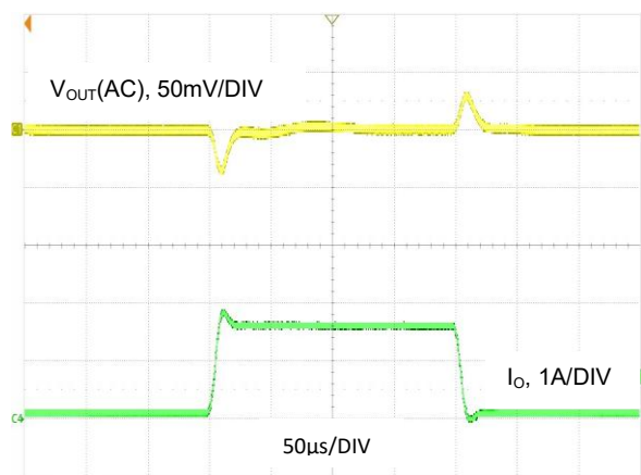
图 15. V OUT = 1.2V, I O = 0.1A 至 1.6A, FPWM 模式
