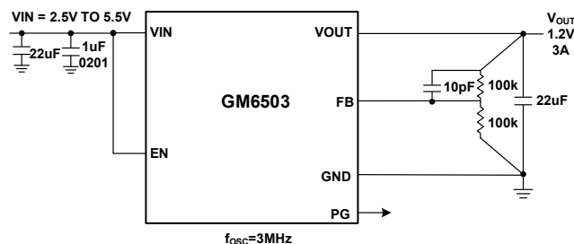
图 1. GM6503 典型应用
