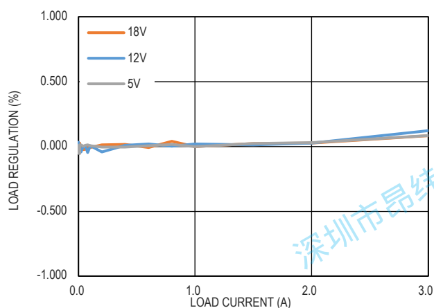
图 6. 输出电压负载调整率, V_{OUT} = 3.3V
