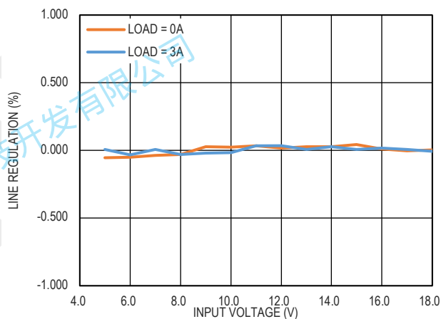
图 7. 输出电压线调整率, V_{OUT} = 3.3V
