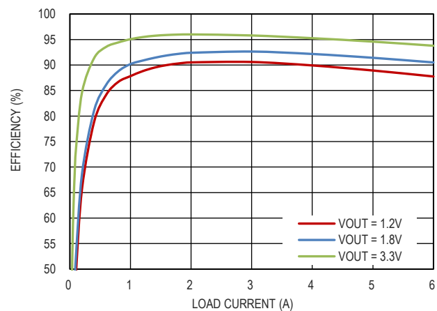
图 12. 效率曲线, V_{IN} = 5V , F_{SW} = 4MHz , FPWM
