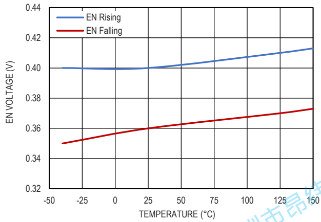
图 19. EN 阈值和温度的关系
