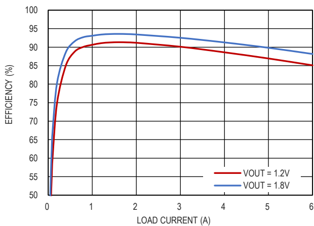
图 9. 效率曲线, V_{IN} = 3.3V , F_{SW} = 2MHz , FPWM
