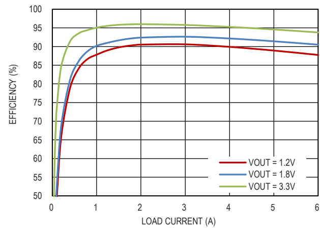
图 10. 效率曲线, V_{IN} = 5V , F_{SW} = 2MHz , FPWM
