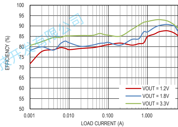
图 8. 效率曲线, V_{IN} = 5V , F_{SW} = 4MHz , 低功耗模式
