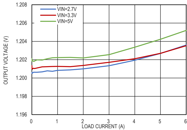
图 17. 输出电压负载调整率, V_{OUT} = 1.2V
