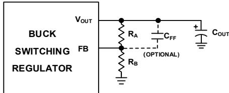
图 29. 反馈电阻网络
