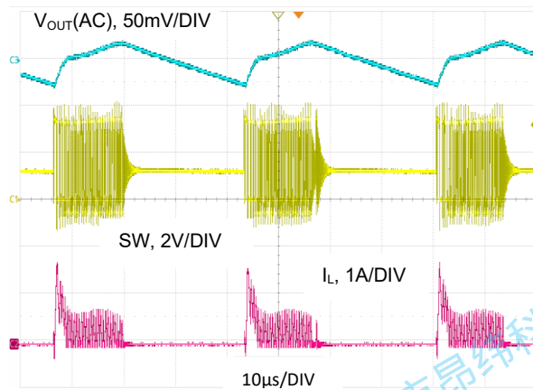
图 25. V_{OUT} = 1.2V , I_O = 10mA , 低功耗模式
