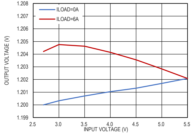
图 18. 输出电压线调整率, V_{OUT} = 1.2V
