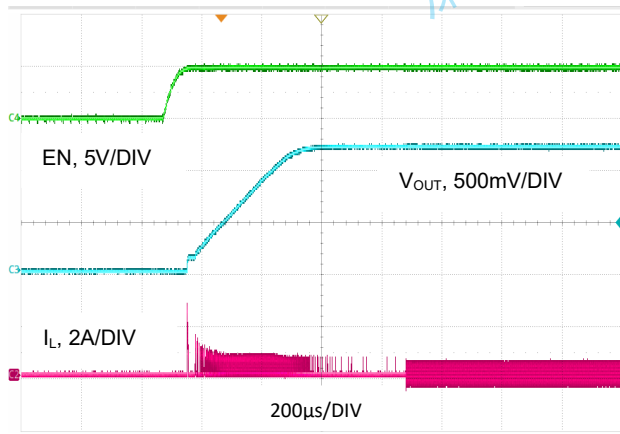
图 21. 启动波形, V_{OUT} = 1.2V , I_O = 10mA
