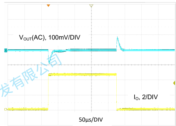
图 26. V_{OUT} = 1.2V , I_O = 0.1A 至 4.5A , FPWM 模式
