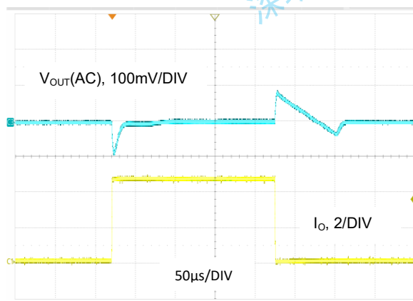
图 27. V_{OUT} = 1.2V , I_O = 0.1A 至 4.5A , PSM 模式
