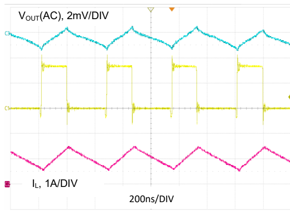
图 23. V_{OUT} = 1.2V , I_O = 1A , FPWM
