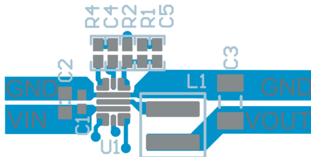
图 30. 推荐的 PCB 布局
