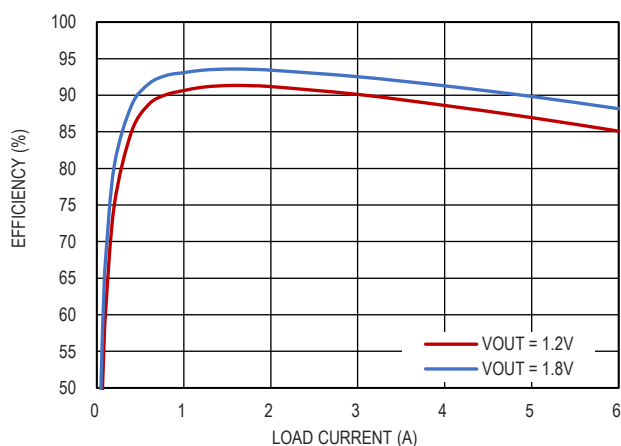
图 11. 效率曲线, V_{IN} = 3.3V , F_{SW} = 4MHz , FPWM
