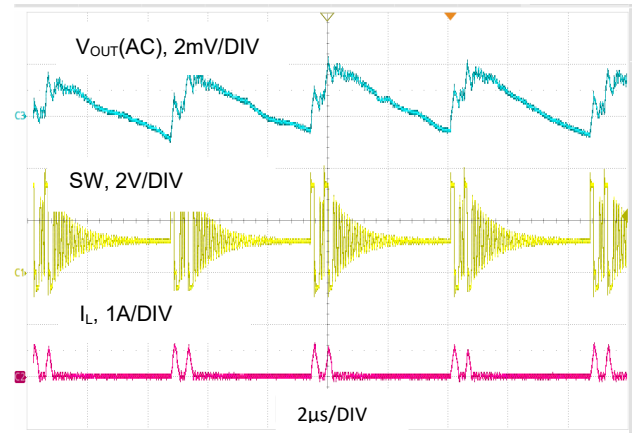
图 24. V_{OUT} = 1.2V , I_O = 100mA , PSM 模式
