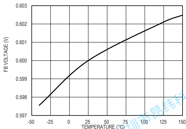
图 13. FB 引脚电压和温度的关系
