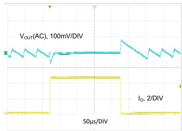
图 28. V_{OUT} = 1.2V , I_O = 0.1A 至 4.5A , 低功耗模式
