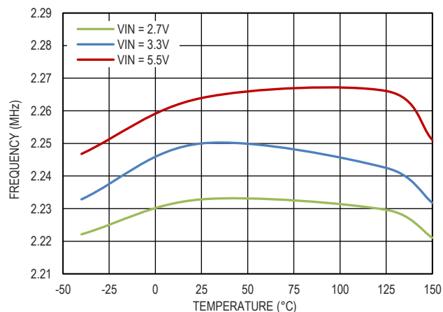
图 16. 频率和温度的关系, R_T 接低
