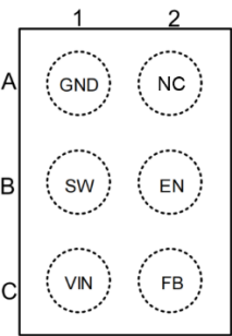
6 引脚 WLCSP
