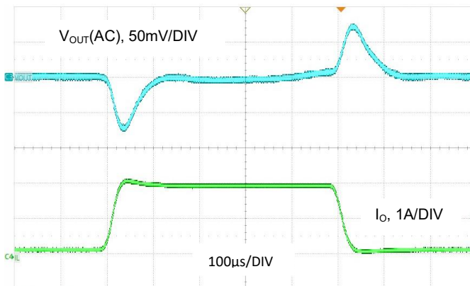
图 18. V_{OUT} = 1.2V , I_o = 0.1A 至 1A , FPWM 模式
