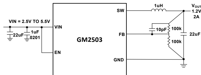
图 1. 1MHz 典型应用
