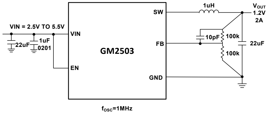
图 21. 1MHz, V_{IN}=3.3V , V_{OUT}=1.2V , I_{LOAD}=2A
