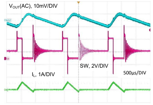
图 16. V_{OUT} = 1.2V , I_O = 100mA , 低功耗模式
