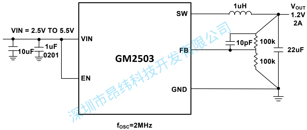
图 22. 2MHz, V_{IN}=3.3V , V_{OUT}=1.2V , I_{LOAD}=2A
