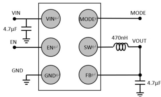
图1. 典型应用
