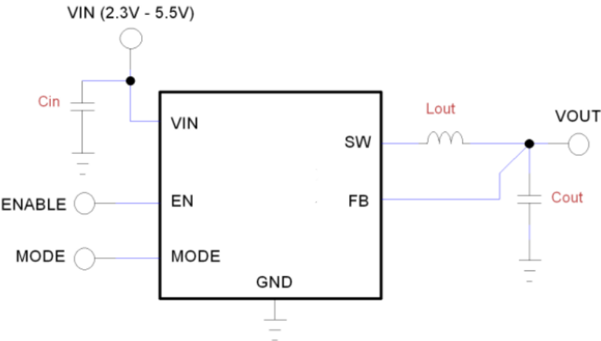
图 44. 应用电路
