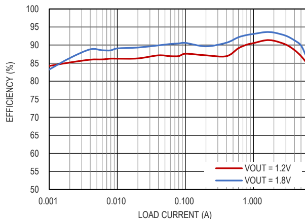
图 6. 效率曲线, V_{IN} = 3.3V , F_{SW} = 2MHz , 低功耗模式
