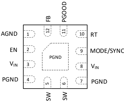
图 4 引脚配置
