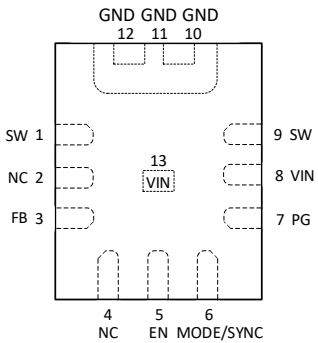
图 5 引脚配置
