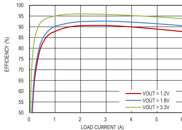
图 11. 效率曲线, V_{IN} = 5V , F_{SW} = 2MHz , FPWM
