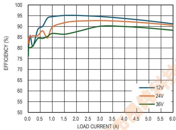
图 8. 效率曲线, V_{OUT} = 5V , L = 3.3uH , F_{SW} = 1MHz
