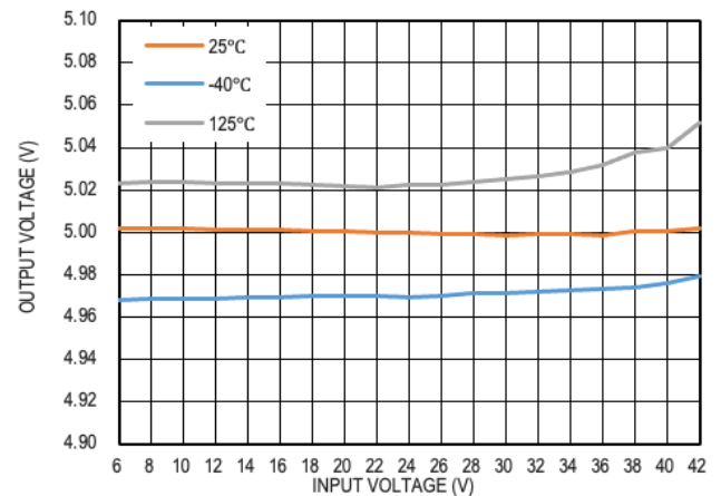
图 11. 输出电压线调整率, V_{OUT} = 5V , 1A
