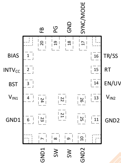
图 3.26 引脚 QFN 封装
