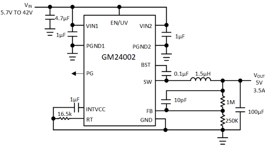
图 20. 2MHz, V_{IN}=12V , V_{OUT}=5V , I_{LOAD}=3.5A
