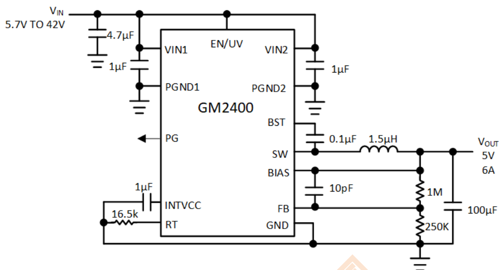
图 18. 2MHz, V_{IN}=12V , V_{OUT}=5V , I_{LOAD}=6A
