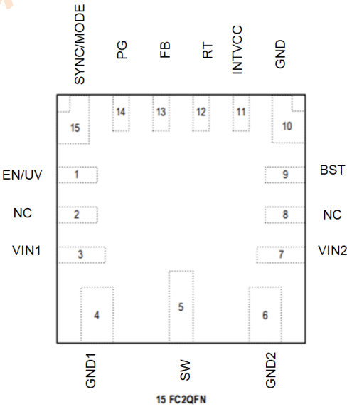
图 4. 15 引脚 QFN 封装
