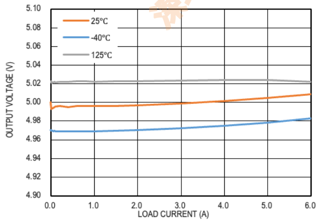
图 10. 输出电压负载调整率, V_{OUT} = 5V
