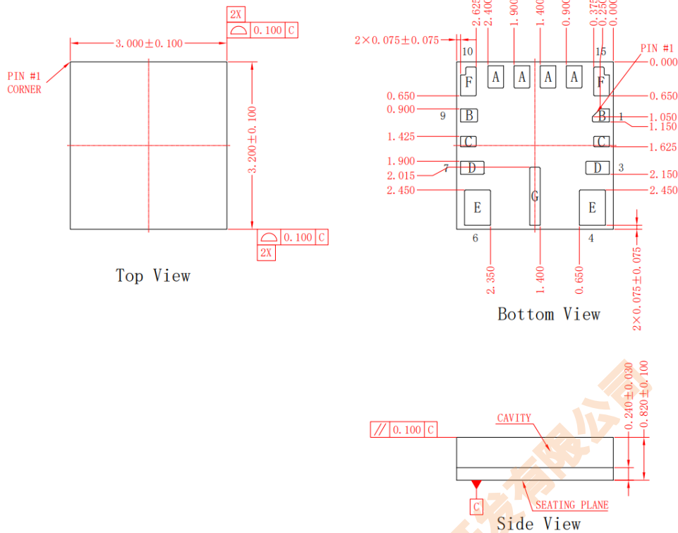
图 22.15 引脚 QFN
