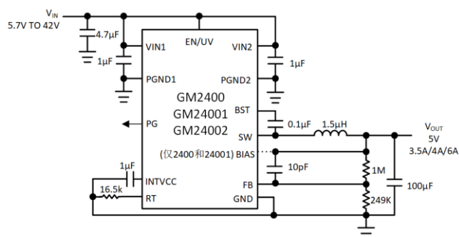
图 1. 2MHz 典型应用
