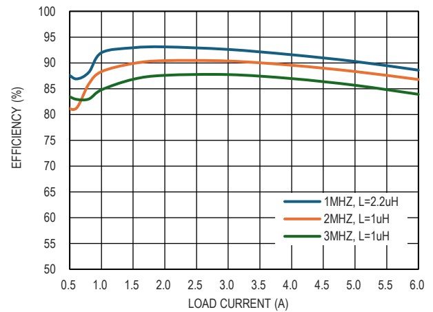
图 7. 效率曲线, V_{IN} = 12V , V_{OUT} = 3.3V
