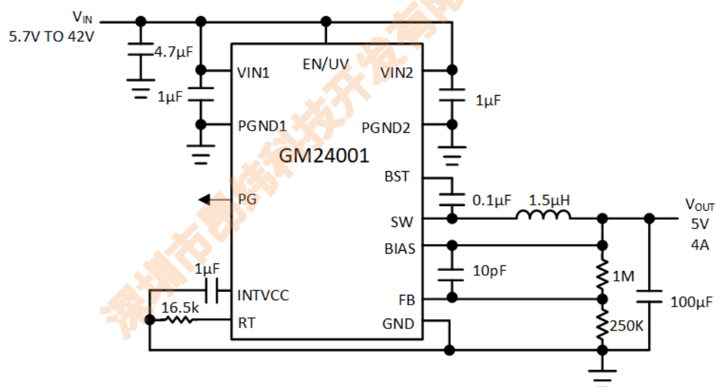
图 19. 2MHz, V_{IN}=12V , V_{OUT}=5V , I_{LOAD}=4A
