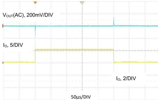
图 15. V_{OUT} = 5V , I_O = 10mA , 低功耗模式
