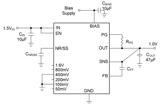
图 1 GM1503-1 典型应用
