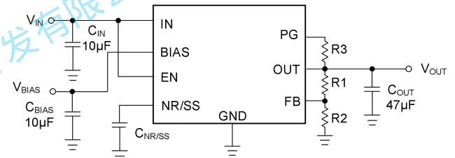
图 2 GM1503-2 典型应用
