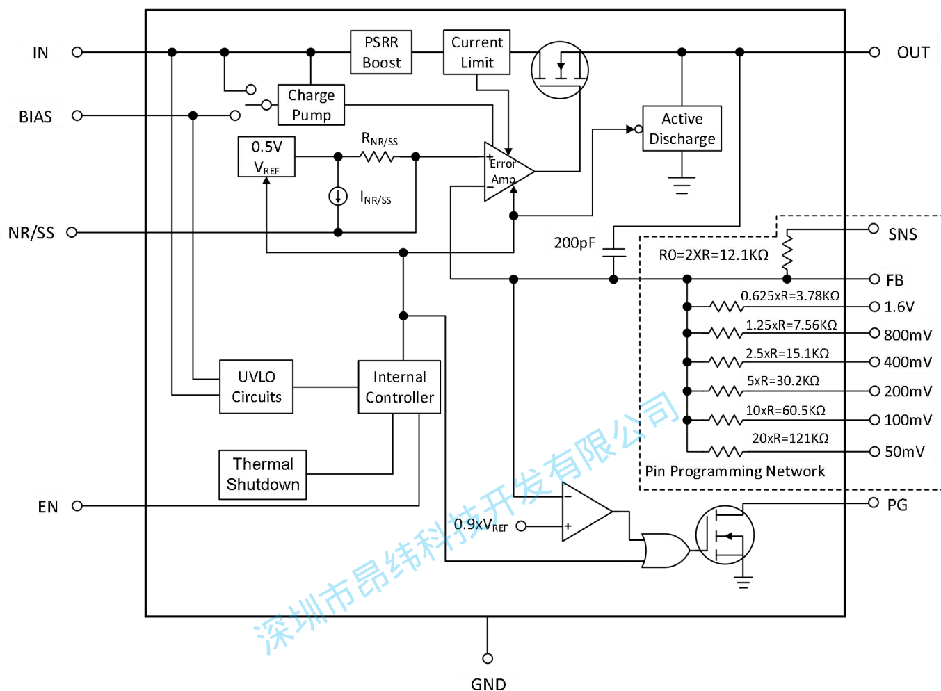
图 3. GM1503-1 方框图
