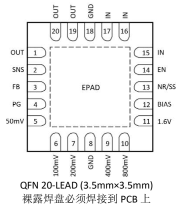
图 5 引脚配置
