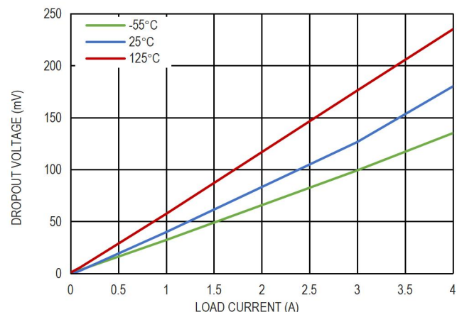
图 12. 压差电压和负载的关系, V_{OUT} = 1.2V , V_{BIAS} = 5V
