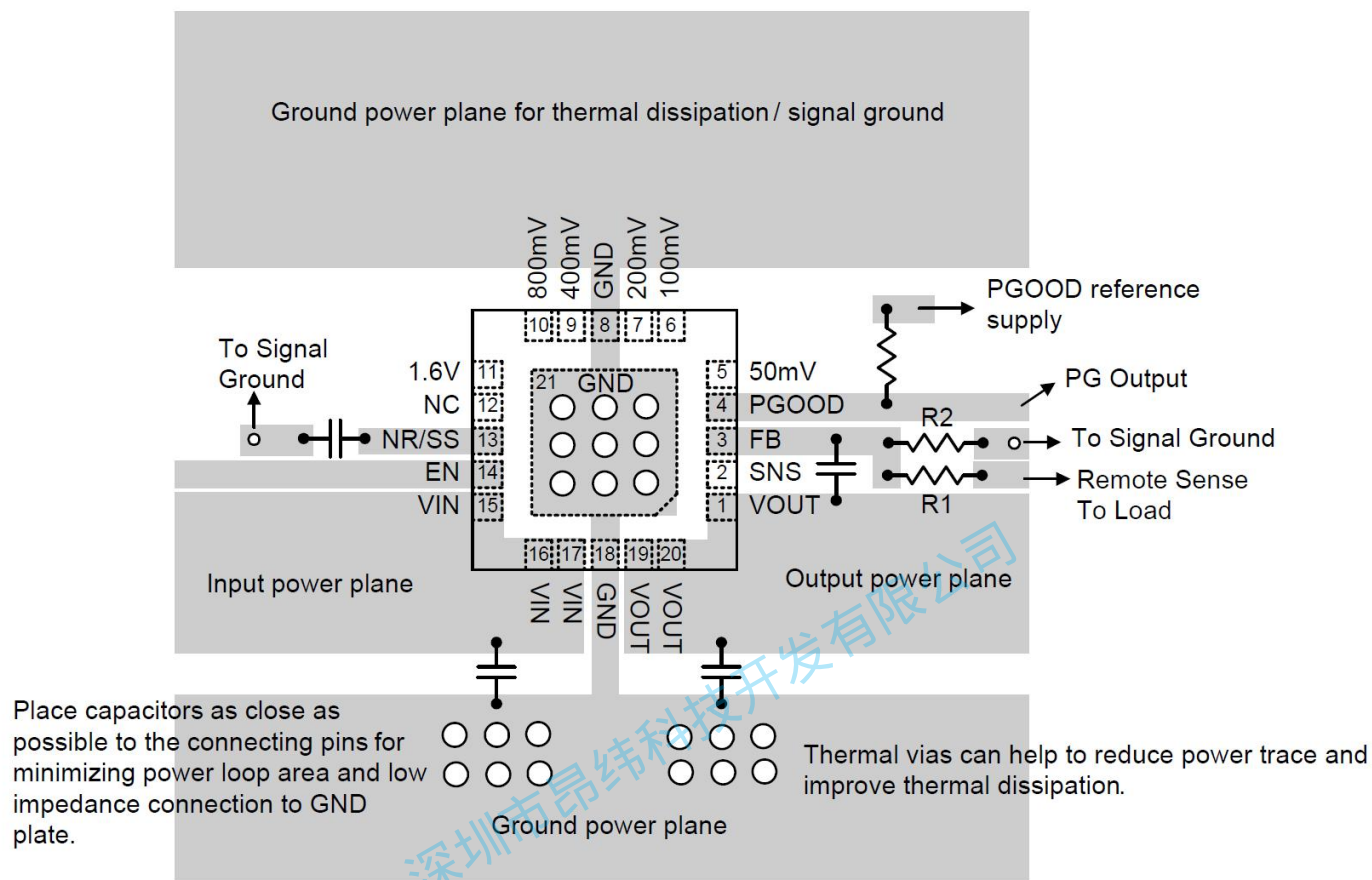
图 29. GM1503-1 布局示例
