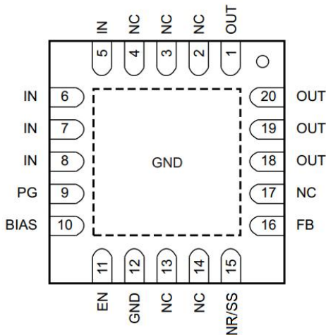
QFN 20-LEAD (5mmx5mm) 裸露焊盘必须焊接到 PCB 上
