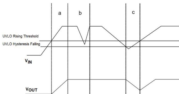
图 26 欠压锁定条件和输出变化
