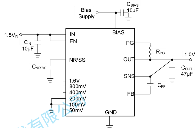
图 25 无需外部电阻的输出电压设置
