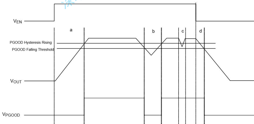
图 27 .PG 触发场景具有不同的运行状态
