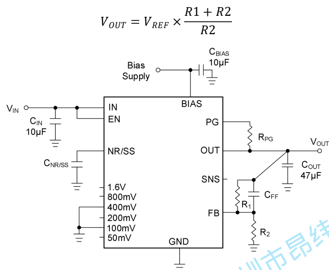
图 24 由外部电阻决定的输出电压
