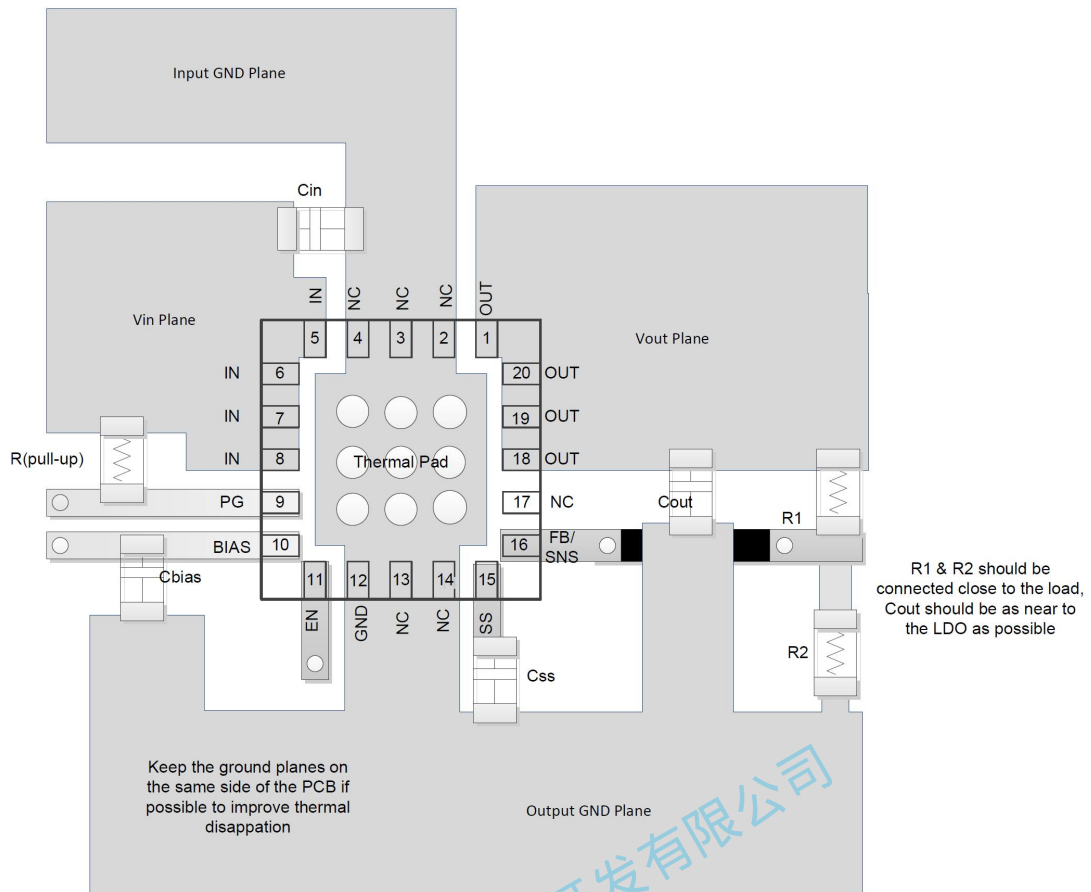
图 30. GM1503-2 布局示例
