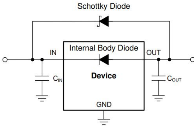
图 28. 反向电流保护应用电路
