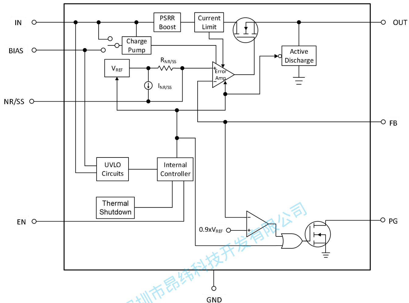
图 4. GM1503-2 方框图
