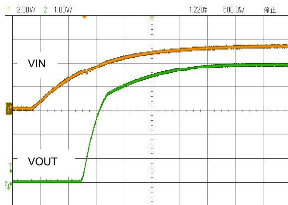
图 16. UVLO 阈值, V_{BIAS} = 5V
