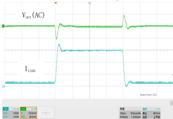
图 23. 负载跳变, V_{IN} = 2.8V , V_{OUT} = 1.8V , I_O = 0.3A 至 3A
