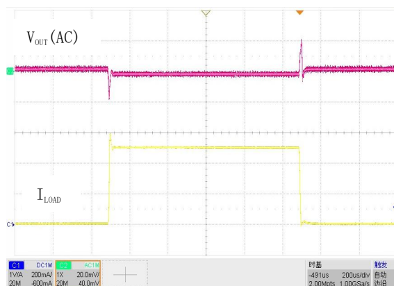
图 21. 负载瞬态响应, V_{IN}=1.2V , V_{OUT}=0.8V , I_{OUT}=1mA to 500mA
