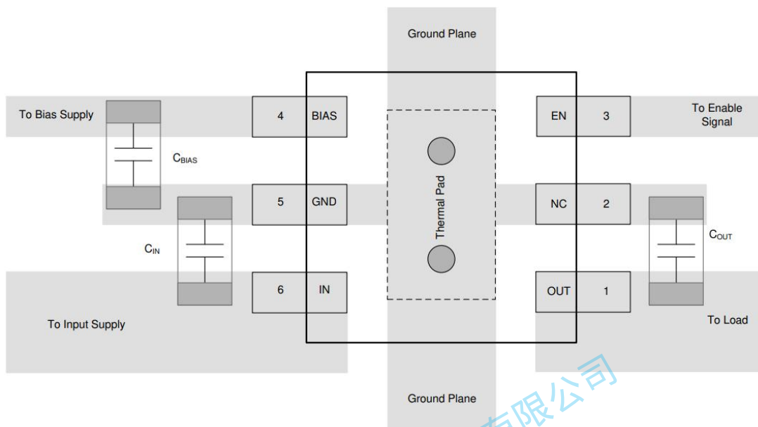
图 22. 版图示例
