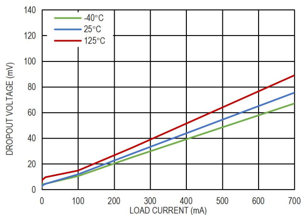
图 4. 压差电压和负载电流的关系, V_{OUT}=0.8V
