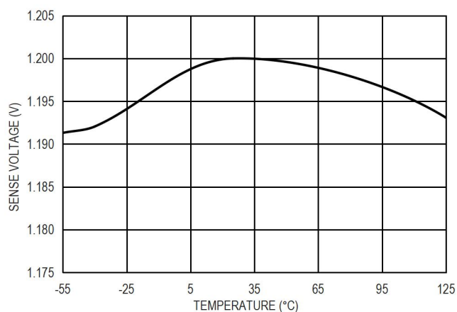
图 12. 1.2V SENSE 引脚电压精度
