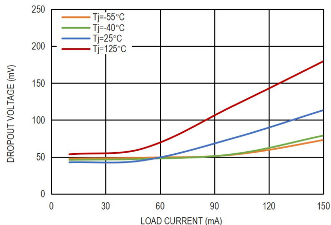
图 6. 5.0V 压差电压和负载电流的关系
