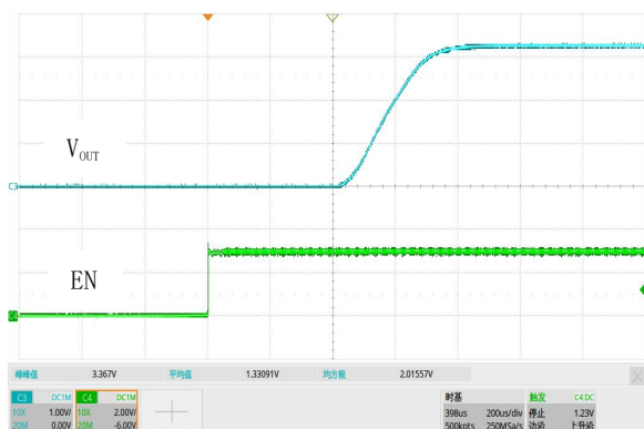
图 21. 软启动, V_{IN}=4.3V , V_{OUT}=3.3V , I_{OUT}=150mA
