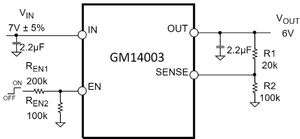
图 27. EN 引脚的典型分压器
