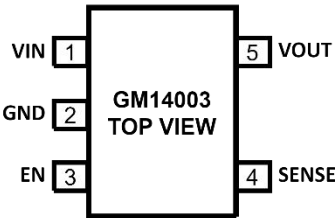
图 3. 5 引脚 SOT 引脚配置
