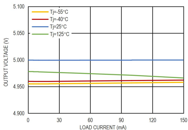
图 11. 5.0V 输出电压和负载电流的关系
