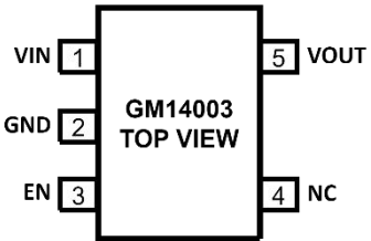
图 4. 5 引脚 SOT 引脚配置
