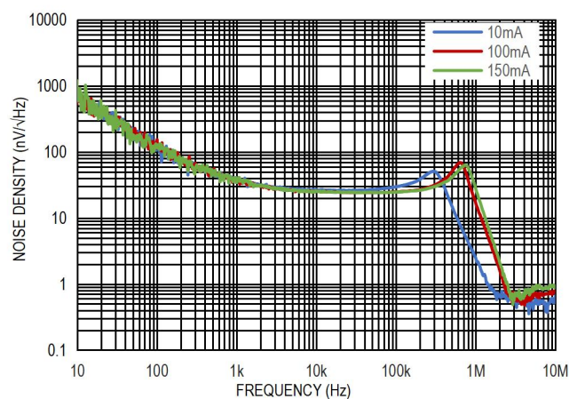
图 16. 输出噪声谱密度, V_{IN}=5V , V_{OUT}=3.3V
