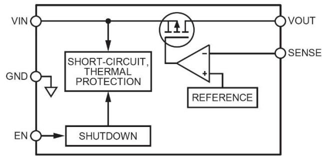
图 23. 内部框图
