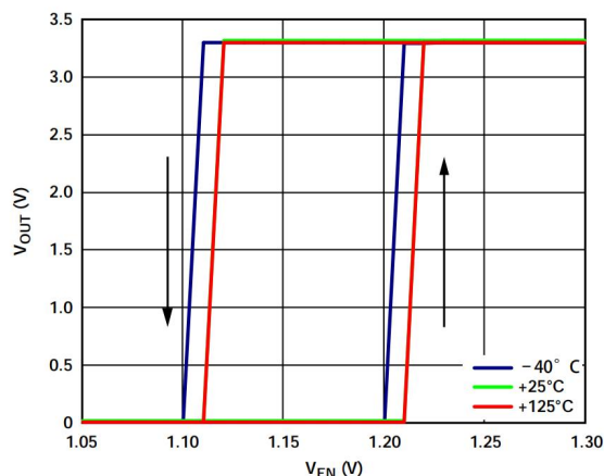
图 26. 对 EN 引脚工作方式的典型 V_{OUT} 响应
