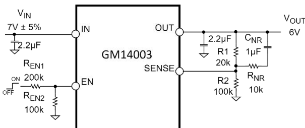
图 28. 噪声优化
