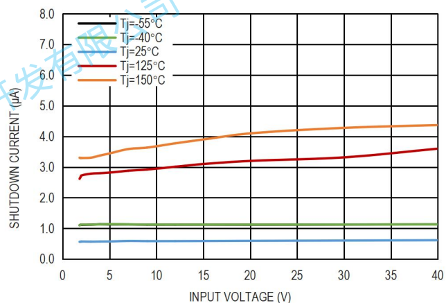
图 8. 关机电流和输入电压的关系
