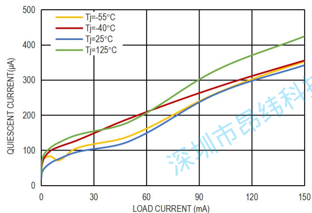
图 7. 静态电流和负载电流的关系, V_{IN} = 4.3V
