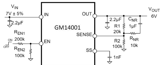
图 29. 噪声优化
