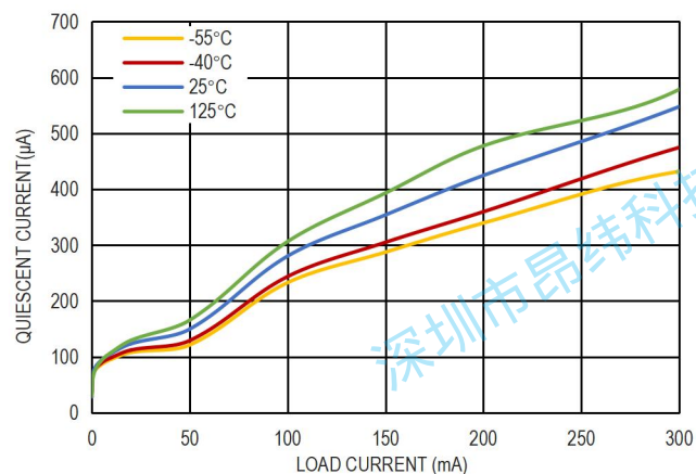
图 10. 静态电流和负载电流的关系, V_{IN} = 4.3V
