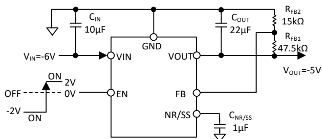
图 1 典型应用
