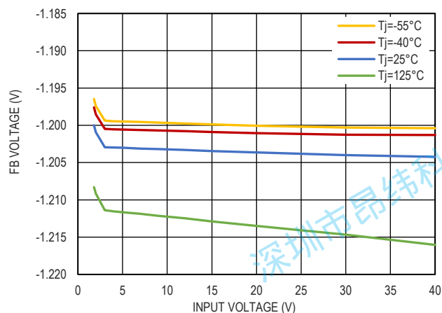
图 5. FB 引脚电压与输入电压的关系
