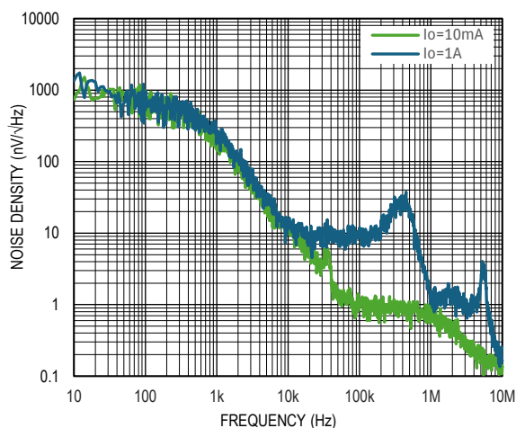
图 9. 噪声谱密度
