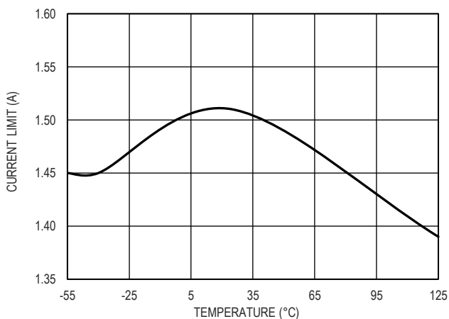
图 14. 限流值和结温的关系
