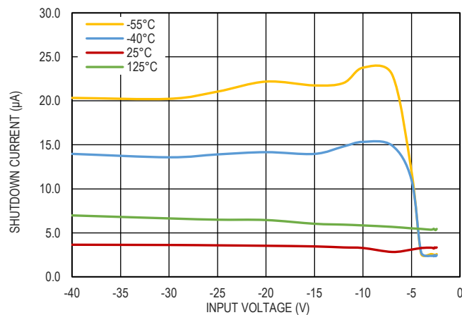
图 7. 关机电流与输入电压的关系
