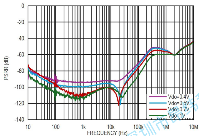
图 19. 电源电压纹波抑制比和压差的关系, I_{OUT}=10mA
