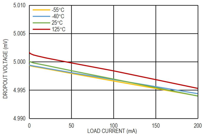
图 10. V_{OUT} = 5.0V 时的负载调整率
