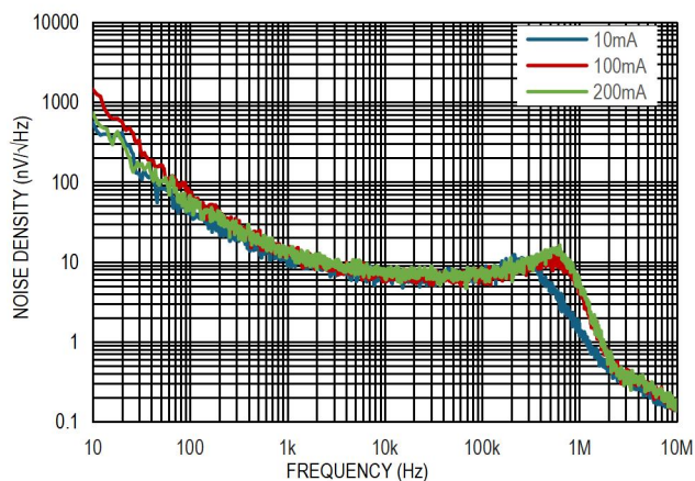
图 18. 输出噪声谱密度, V_{IN}=4.3V , V_{OUT}=3.3V
