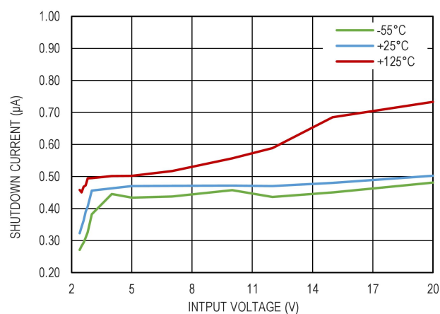
图 12. 停机静态电流和输入电压的关系
