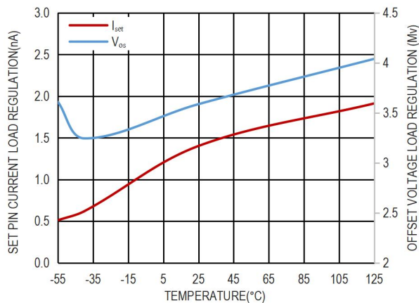
图 9. SET pin 电流、 |V_{OUT} - V_{SET}| 和温度的关系
