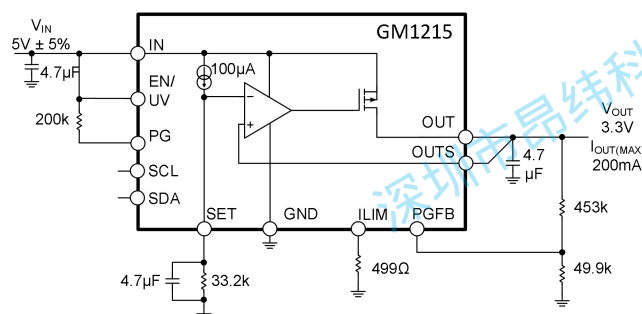
图 23 典型应用
