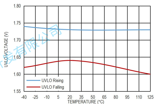
图 14. UVLO 阈值
