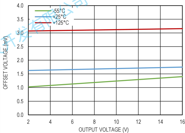
图 8. |V_{OUT} - V_{SET}| 和输出电压的关系
