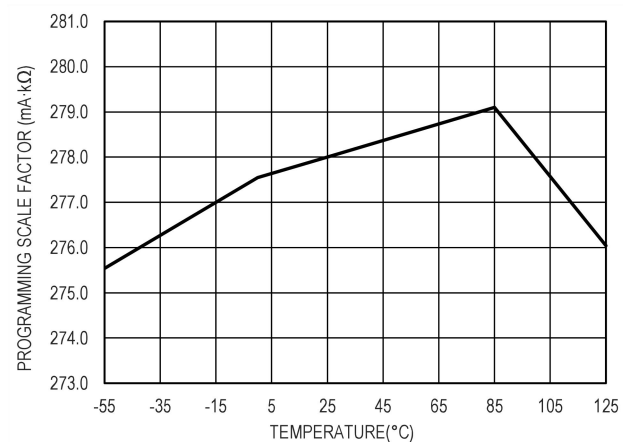
图 16. 输出限流值编程因子
