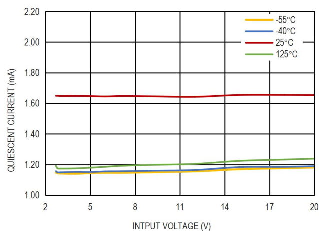
图 11. 静态电流和输入电压的关系, I_{OUT}=1mA
