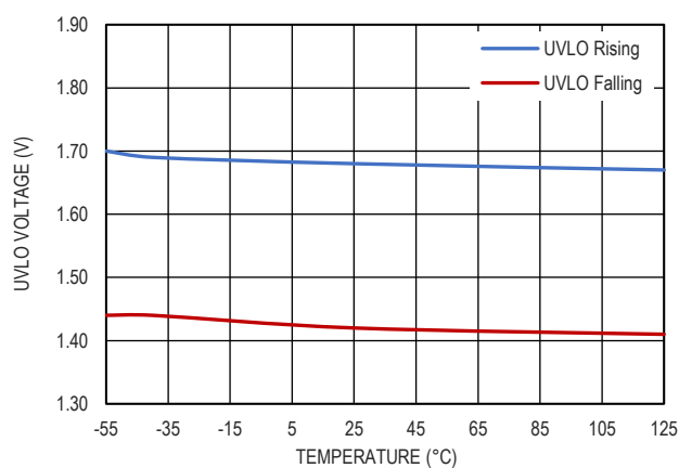
图 17. UVLO 阈值和温度的关系
