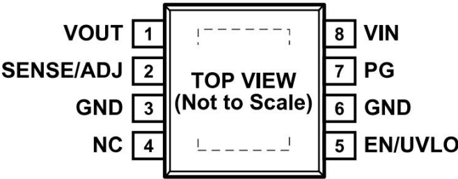
图 5.8 引脚 SOP-8 的引脚配置
