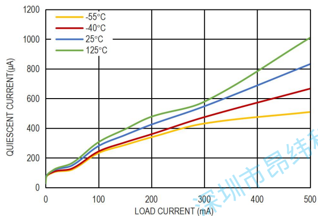
图 8. 静态电流和负载电流的关系, V_{IN}=4.3V
