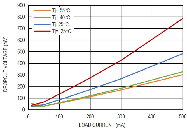
图 6. 3.3V 压差电压和负载电流的关系
