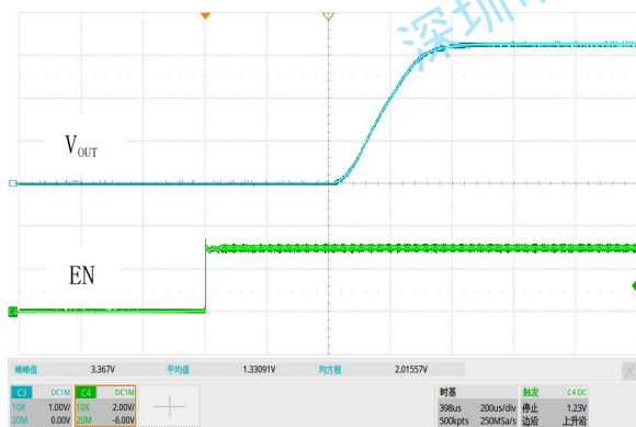
图 22. 软启动, V_{IN}=4.3V , V_{OUT}=3.3V , I_{OUT}=500mA
