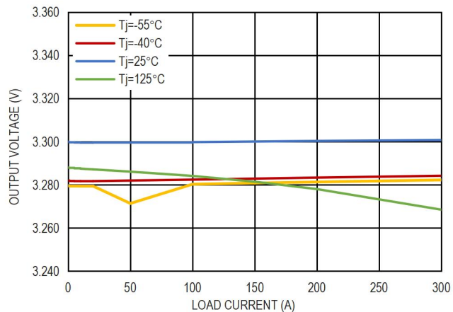
图 11. 3.3V 输出电压和负载电流的关系
