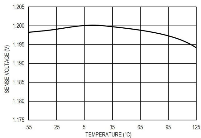
图 13. 1.2V SENSE 引脚电压精度
