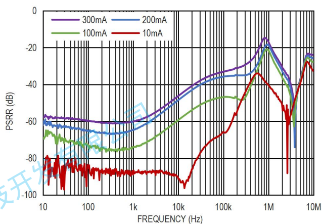
图 21. 电源电压纹波抑制比与负载的关系, V_{OUT}=5.0V
