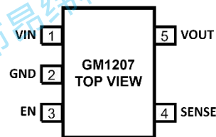
图 4.8 引脚 SOT-23 的引脚配置
