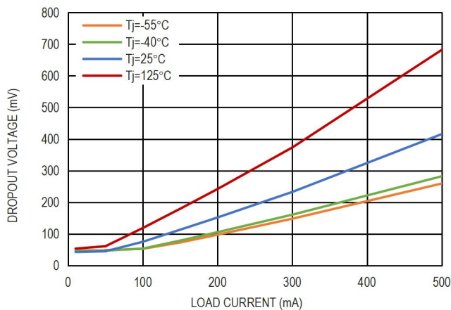
图 7. 5.0V 压差电压和负载电流的关系
