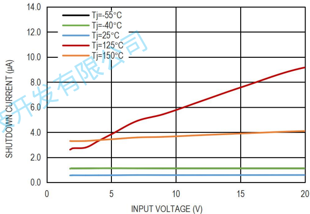
图 9. 关机电流和输入电压的关系
