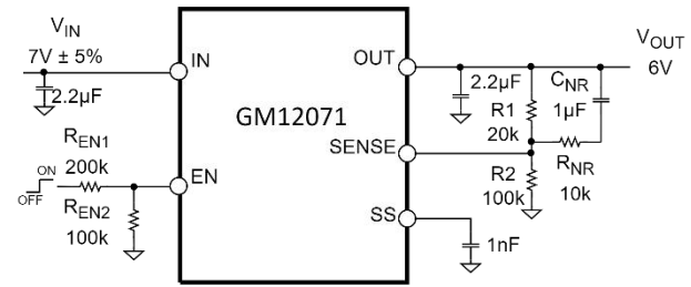
图 29. 噪声优化
