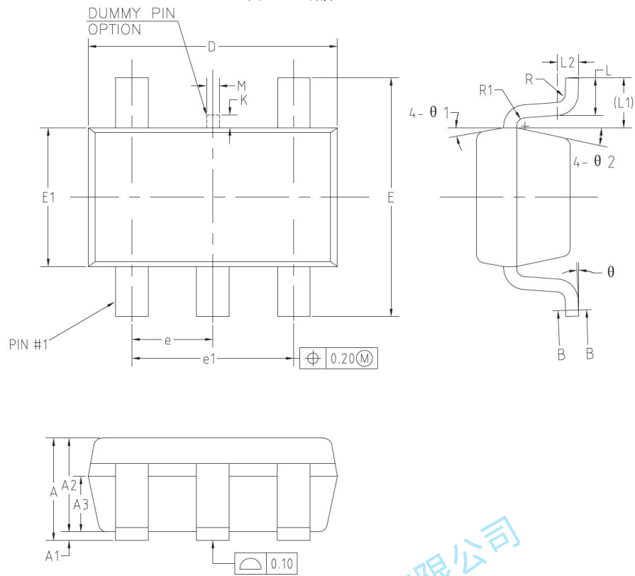
图 30.6 引脚 DFN-6
