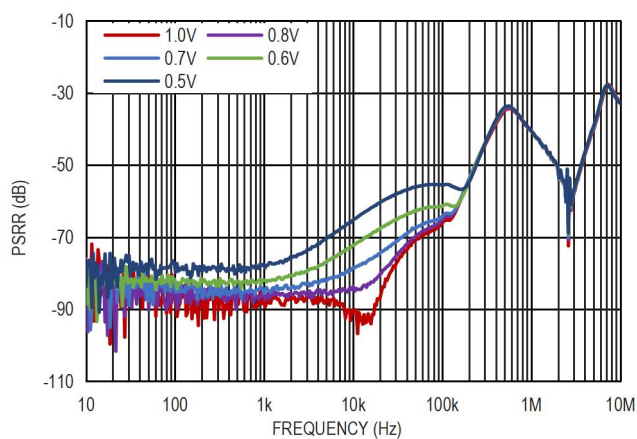
图 19. 电源电压纹波抑制比与压差的关系, V_{OUT}=5.0V
