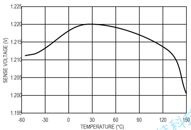
图 14. 1.22V SENSE 引脚电压精度
