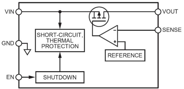
图 24. 内部框图
