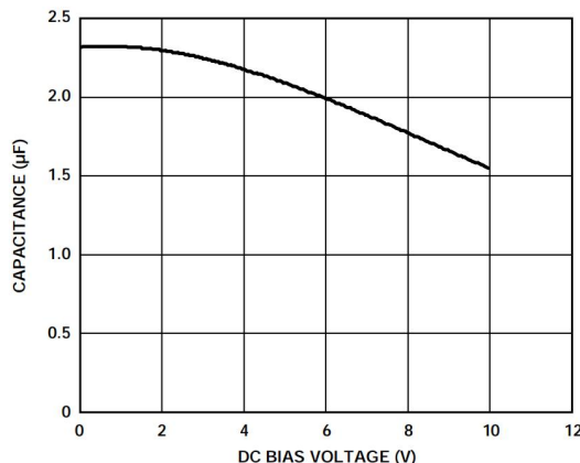
图 27. 电容与电压关系特性
