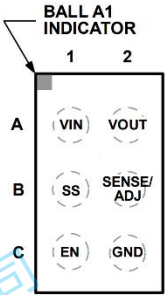
图 6.6 引脚 WLCSP 引脚配置
