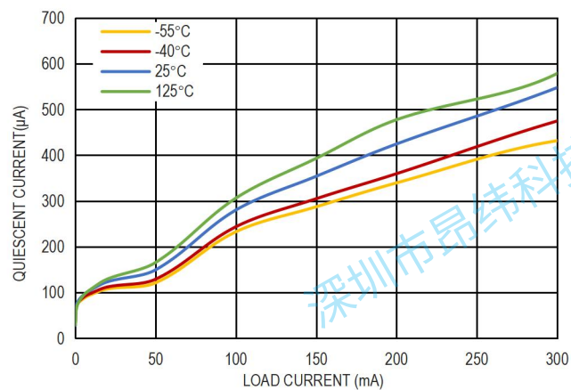
图 9. 静态电流和负载电流的关系, V_{IN}=4.3V
