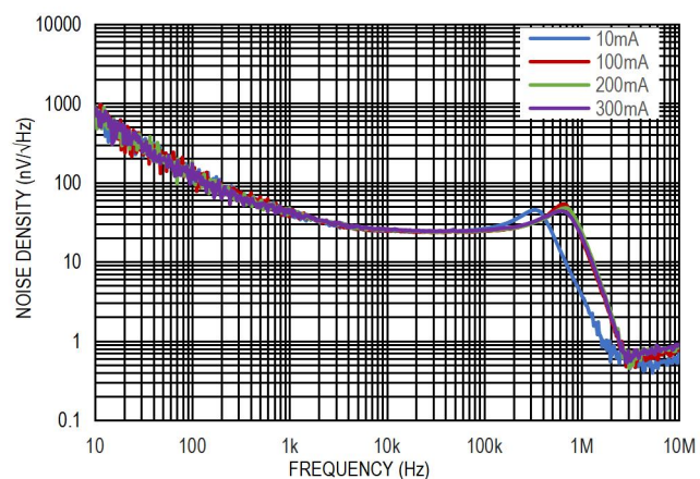
图 18. 输出噪声谱密度, V_{\text{IN}}=5\text{V} , V_{\text{OUT}}=3.3\text{V}
