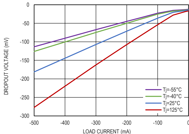
图 8. 压差电压和负载电流的关系
