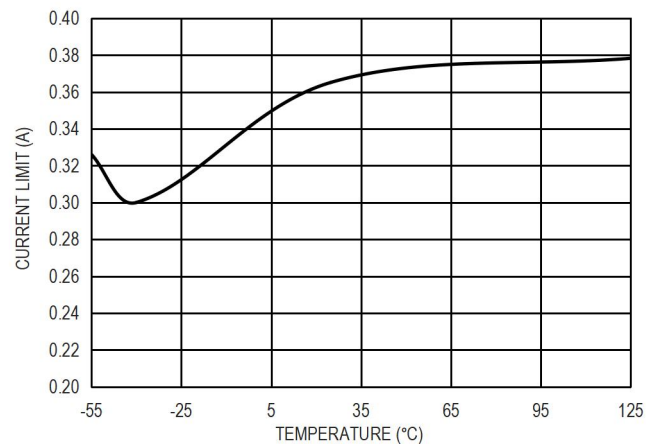
图 15. 限流值和结温的关系
