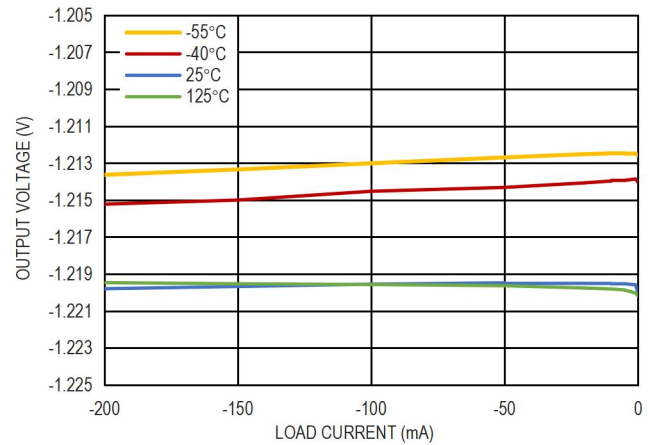
图 5. ADJ 引脚电压与 vs. 负载电流的关系
