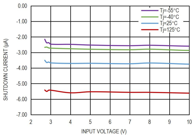
图 8. 静态电流与输入电压的关系
