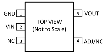
图 3. SOT-23 引脚配置(顶视图)
