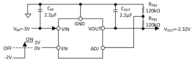
图 20. 设置可调输出电压
