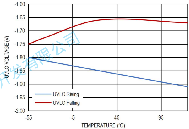
图 13. UVLO 阈值和结温的关系
