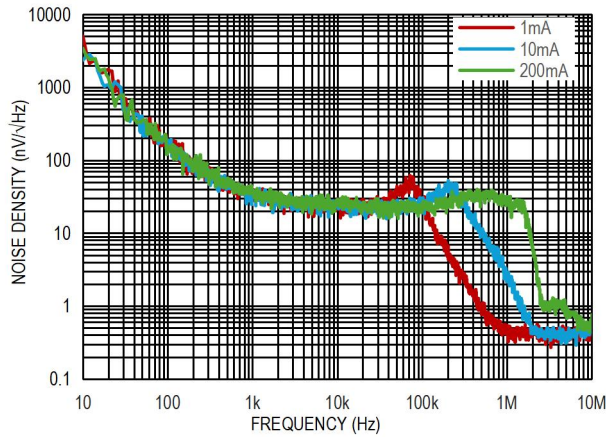
图 10. 噪声谱密度
