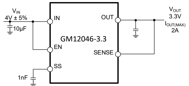
图 1 典型应用
