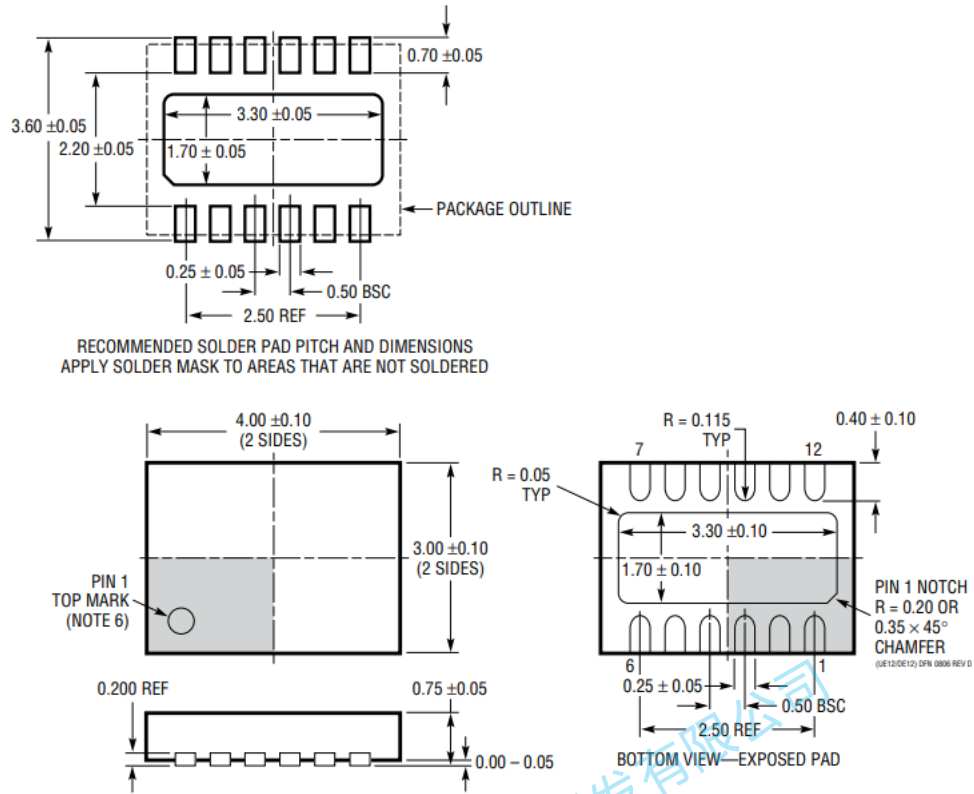
图 22. 16 引脚 TSSOIC
