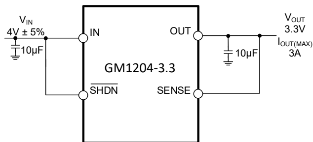
图 1 典型应用
