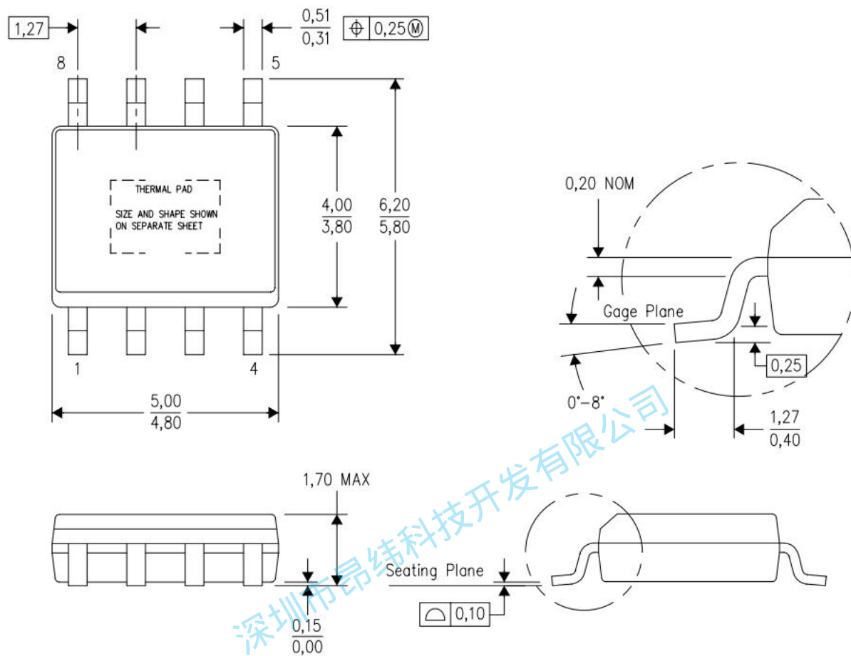
图 18.8 引脚 PSOP
