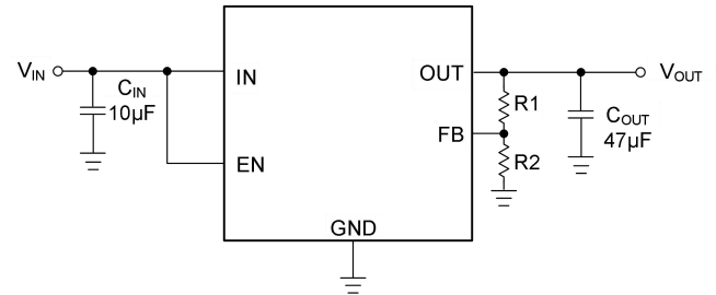
图 1 典型应用
