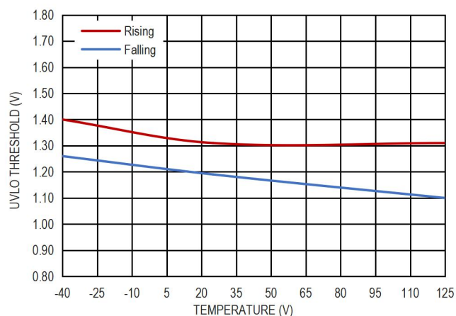
图 9. UVLO 阈值
