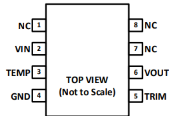
图 2. 8 引脚 SOIC
