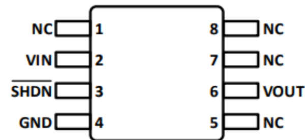
图 1. 8 引脚 MSOP
